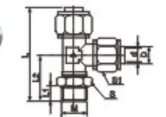
FN-Y 三通边部终端管接头 360° 旋转
