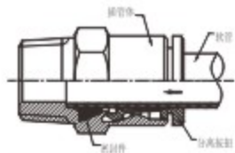
FCR-终端接头 FCR-Male stud
