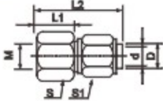
FN-B 直角终端内螺接头 FN-Female stud
